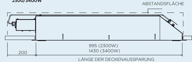
Einbausatz für niedrige Deckenhöhen 2300/3400W
