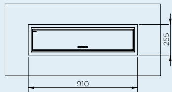
DECKENVERTIEFUNG FÜR 2300-W-RAHMEN
