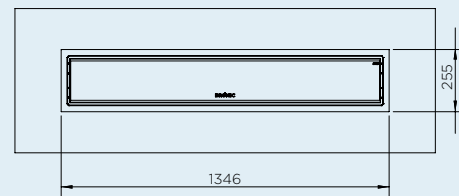
MINDESTVERTIEFUNG OPTION 2 2300/3400W
