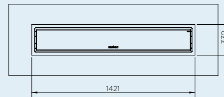
MINDESTVERTIEFUNG FÜR 4500W
