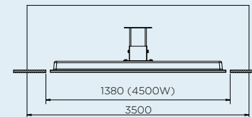
MINDESTVERTIEFUNG FÜR 4500W
