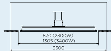
MINDESTVERTIEFUNG OPTION 2 2300/3400W
