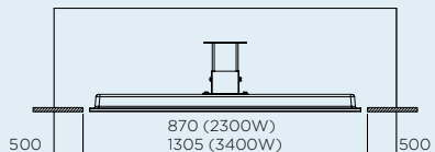
MINDESTVERTIEFUNG OPTION 1 2300/3400W
